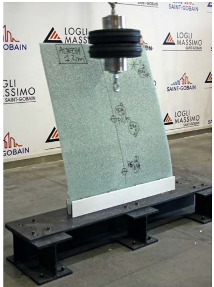
Post-rupture avec intercalaire rigide
