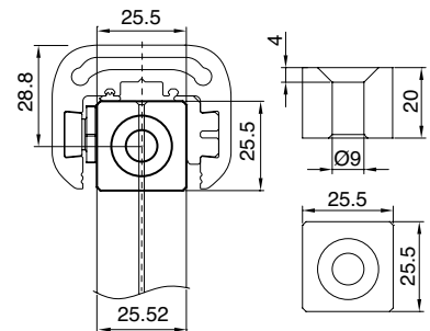
Installation pour verre 12+12 CORLM39B
