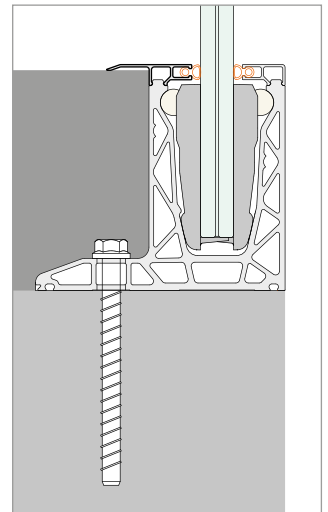
Exemple d'installation Defender DF88DK avec profil de finition de sol DF8801 et profil de finition DF105
